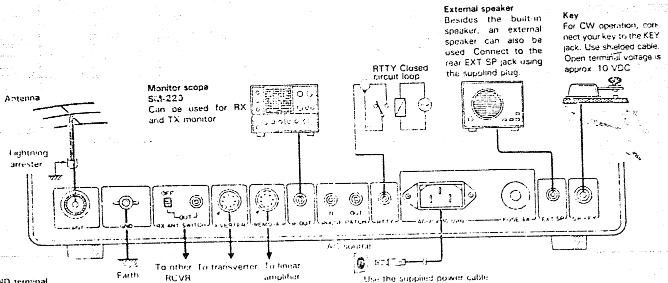
Fig. 3-2 Come eseguire i collegamenti del microfono, del tastatore e degli altri.
