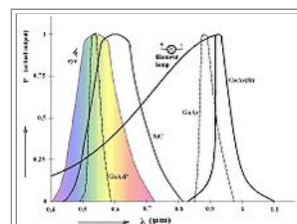
Spettro luminoso di vari LED, messi a confronto con lo spettro visivo dell'occhio umano e della lampada ad incandescenza
