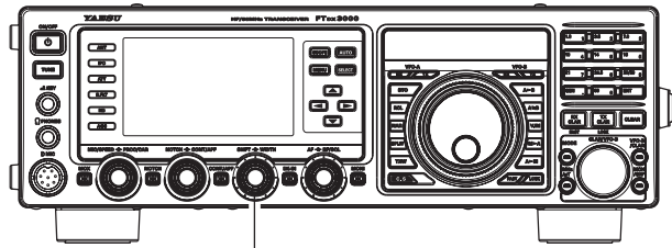
[WIDTH] Knob
