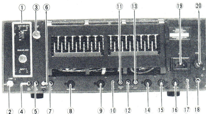
Pannello posteriore.
