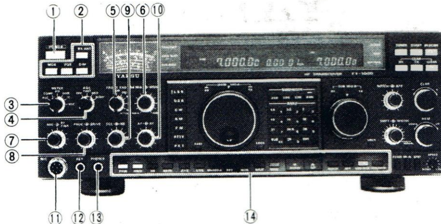
Pannello frontale
