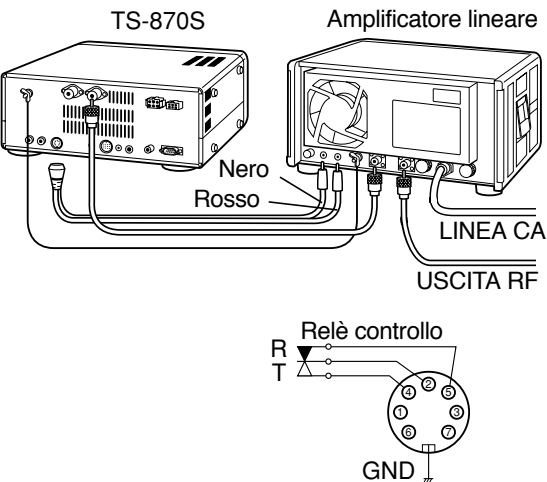
Connettore REMOTE (Vista pannello posteriore)
