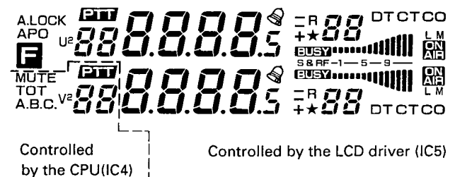
Fig. 16 Display LCD
