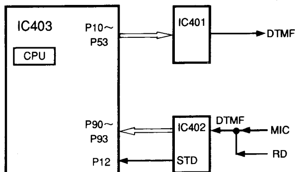
Fig. 10 DTMF encode/decode circuit
