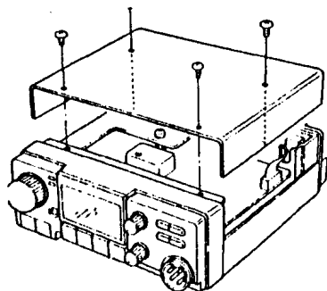
• Rimozione del cofano superiore
