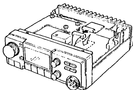
• Installazione dell'UT-40
