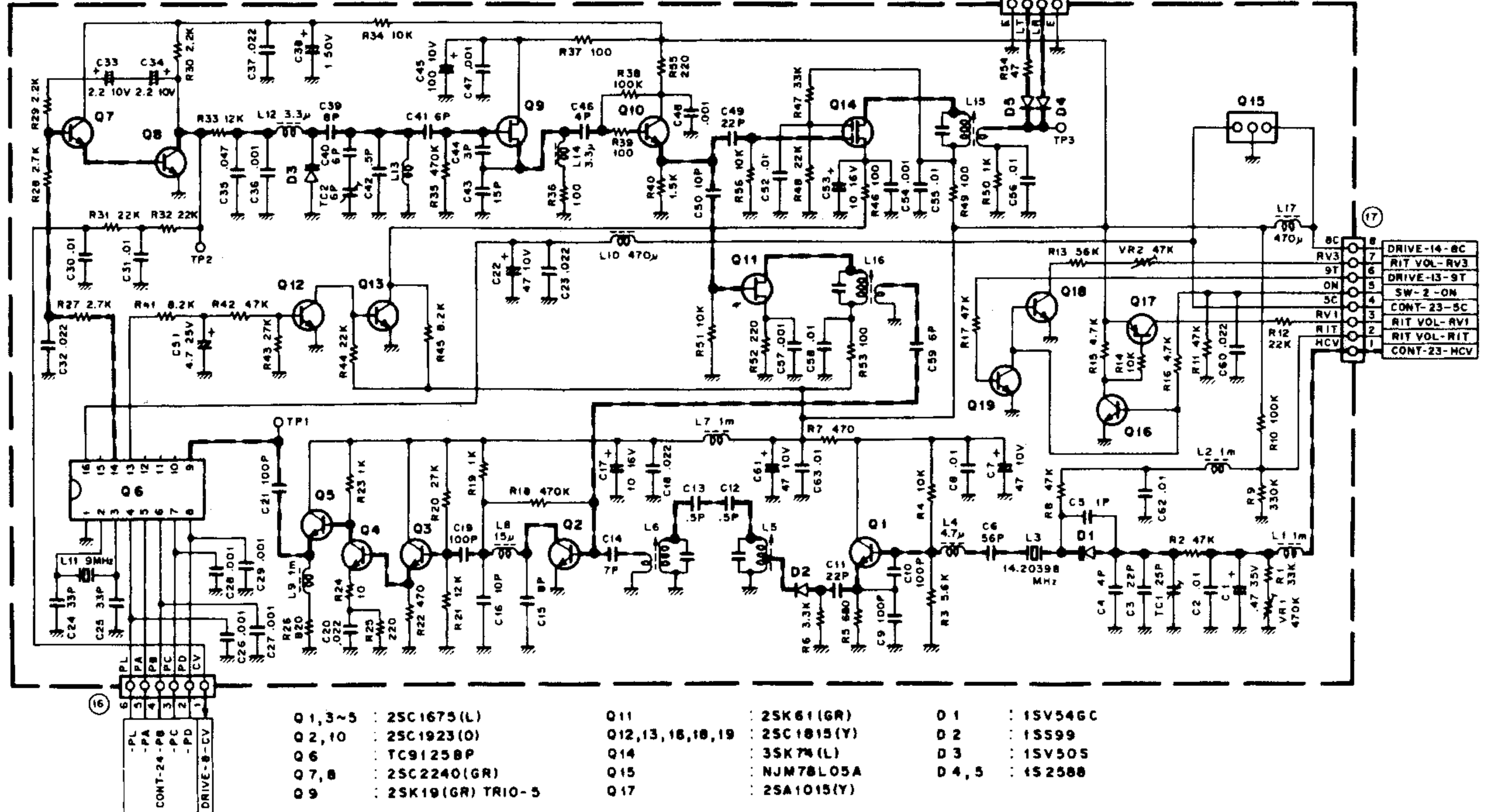
PLL UNIT (X50-1860-00)
