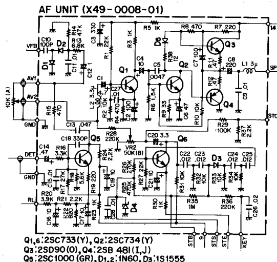
Fig. 19 AF Board
