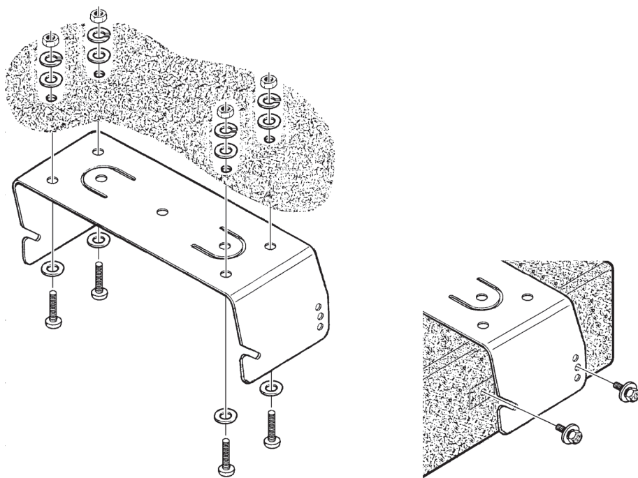
Installazione con staffa MMB-36
