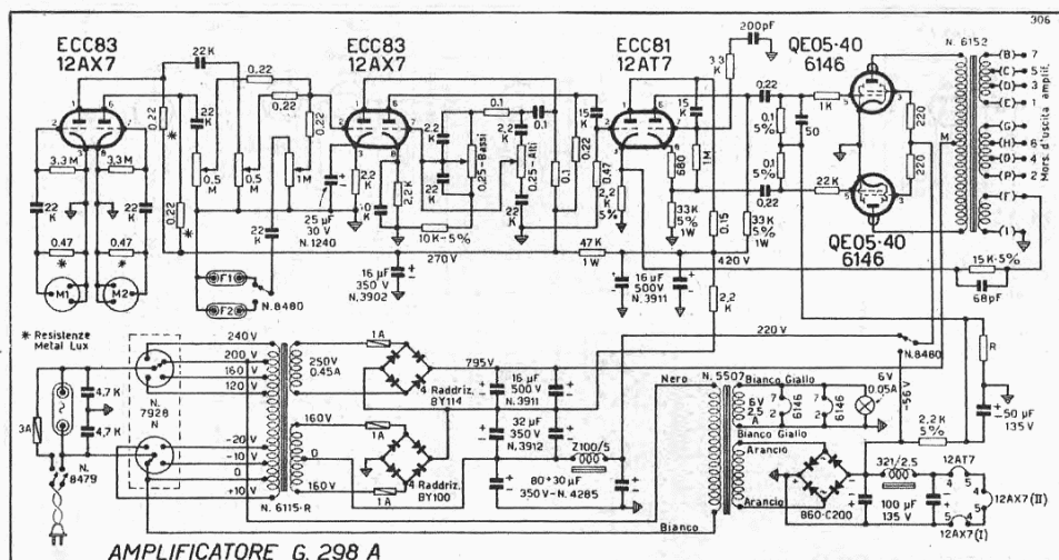
AMPLIFICATORE G. 298 A
