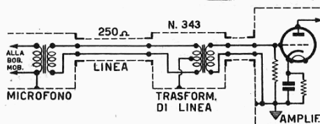
Collegamento di un microfono dinamico
