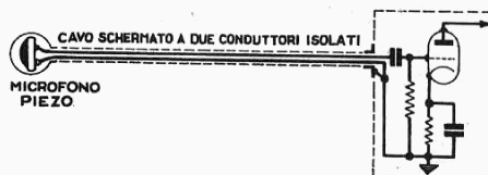
Collegamento di un microfono piezoelettrico
