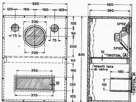
Fig. 2 - Altro modello di mobile « bass-reflex ». Pareti in legno d'abeto, spessore \text{cm } 2 \div 3 . L'imbottitura, da farsi sulla sola parete di fondo, è formata con lana di vetro com'è detto per il mobile della fig. 1. Il mobile è diviso all'interno in due parti uguali mediante un diaframma di materiale foncoassorbente forato (con 100 fori \varnothing 3 \text{ mm} per decimetro quadrato). Tale diaframma potrà essere richiesto a qualche ditta che tratta materiali di questo genere (la nostra Casa per ragioni di correttezza non dà indirizzi). La finestra inferiore è munita di una appendice tubolare di sezione rettangolare posta all'interno del mobile, come mostra la figura, e chiusa nella parte esterna con un diaframma di materiale foncoassorbente forato come il diaframma mediano interno.
