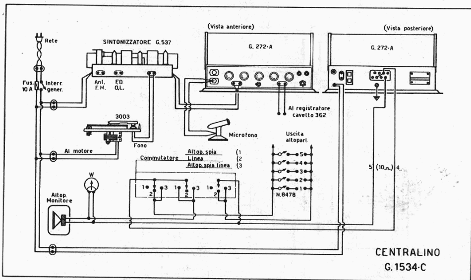
Schema generale del G 1534-C
