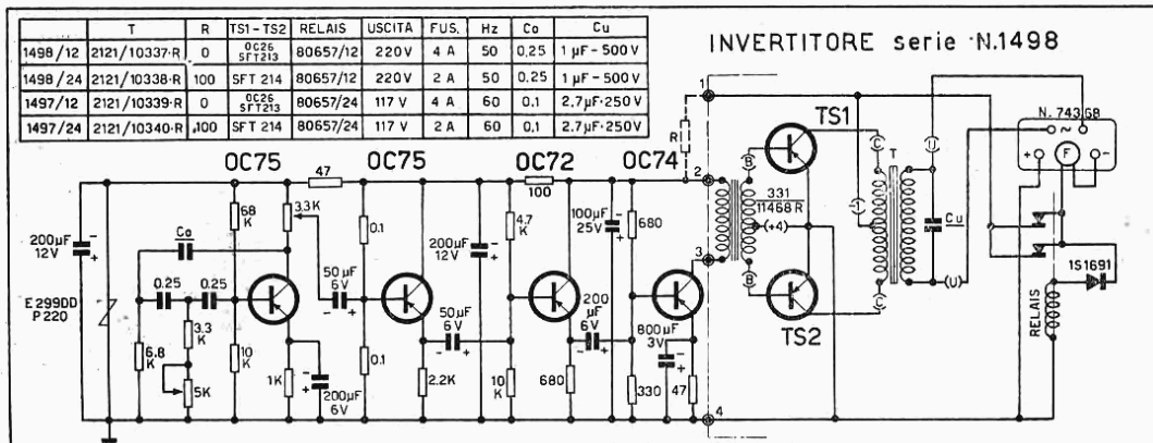
Schema elettrico degli invertitori 20 VA 12 e 24 V.
