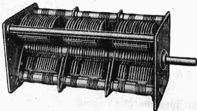
Condensatore variabile triplo della Serie 770
