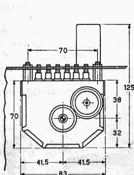
FISSAGGIO AL TELAIO
