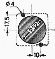
Foratura telaio
