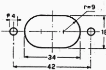
FORATURA TELAIO
