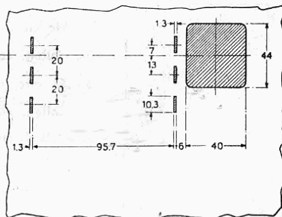
FORATURA DEL TELAI
