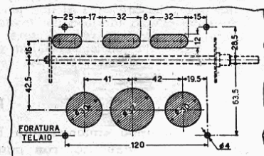
Foratura del telaio
