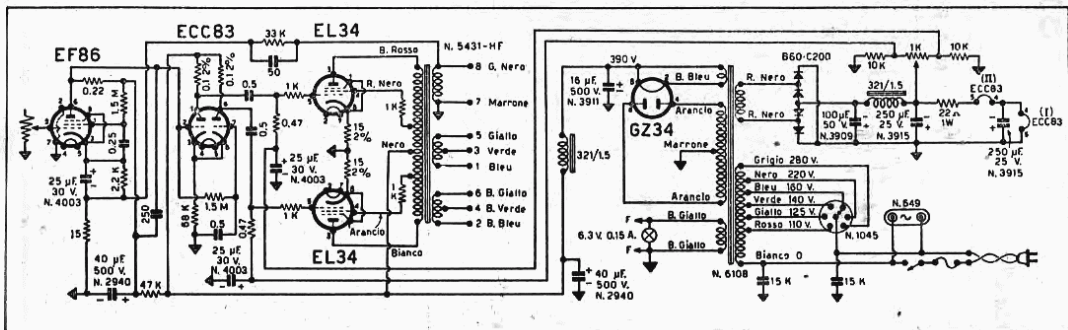
Esempio d'impiego di un trasformatore ad Alta Fedeltà.
