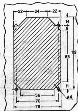
FORATURA TELAIO
