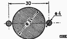
Foratura chassis Mod. 1044 - 45 - 46.
