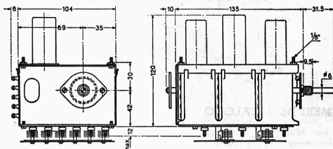
Dimensioni d'ingombro
