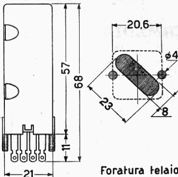
Dati di ingombro e foratura del telaio.
