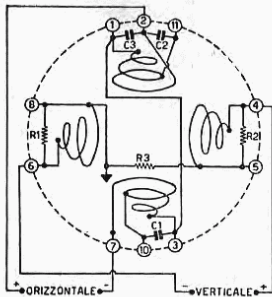
Schema del N. 7215/D
