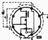
Attacchi allo zoccolo dei vibratori serie N. 1458 (visti di sotto).
