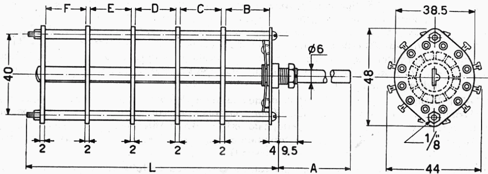
Dati d'ingombro dei commutatori serie 2000.
