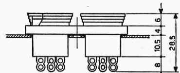
Foratura chassis Mod. 1044 - 45 - 46.
