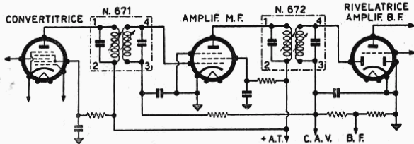
Esempio tipico di impiego: numerazione e corrispondenza dei terminali.
