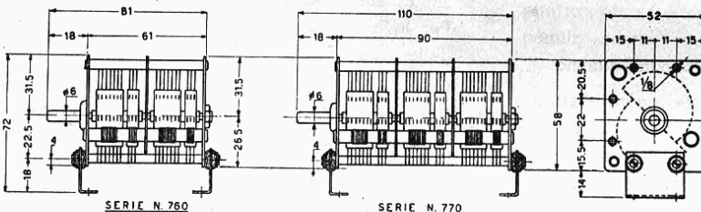
Condensatore variabile triplo della Serie 770
