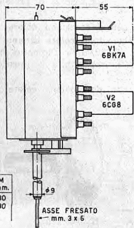
FISSAGGIO AL TELAIO
