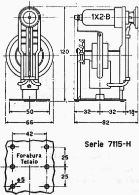
Dimensioni d'ingombro e foratura del telaio dei trasformatori N. 7115-H, N. 7116-H, N. 7117-H.
