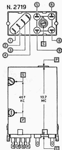
TRASFORMATORE A FI N. 2719
