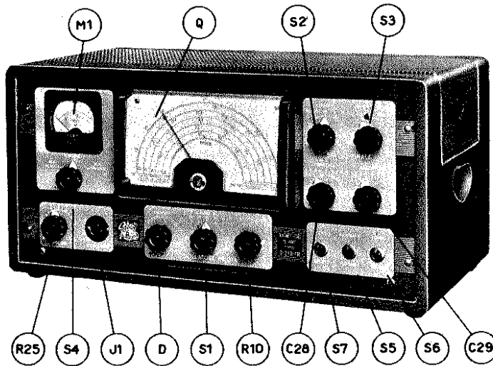
Fig. 4.1 - Vista frontale e nomenclatura organi di comando.
