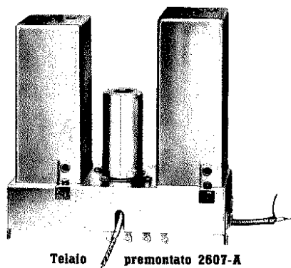
Telaio premontato 2607-A
