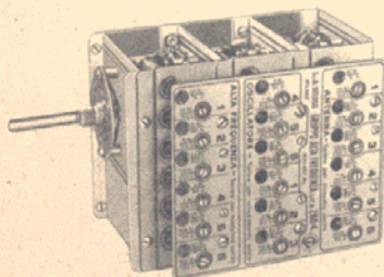
Gruppo per Alta Frequenza N. 2604
