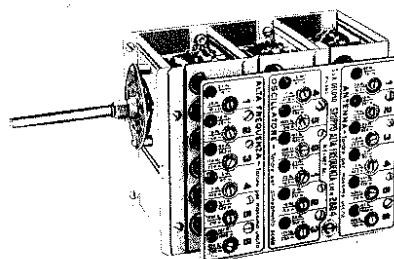
Gruppo di Alta Frequenza Mod. 2616
