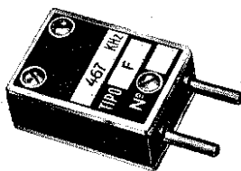
Cristallo di quarzo N. 8449 con supporto
