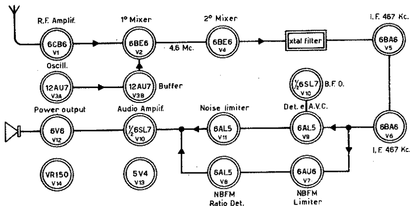
Schema di principio con indicazione delle valvole e della loro funzione.
