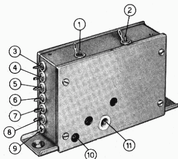
Fig. 3 a - Sintonizzatore n. 12/56
