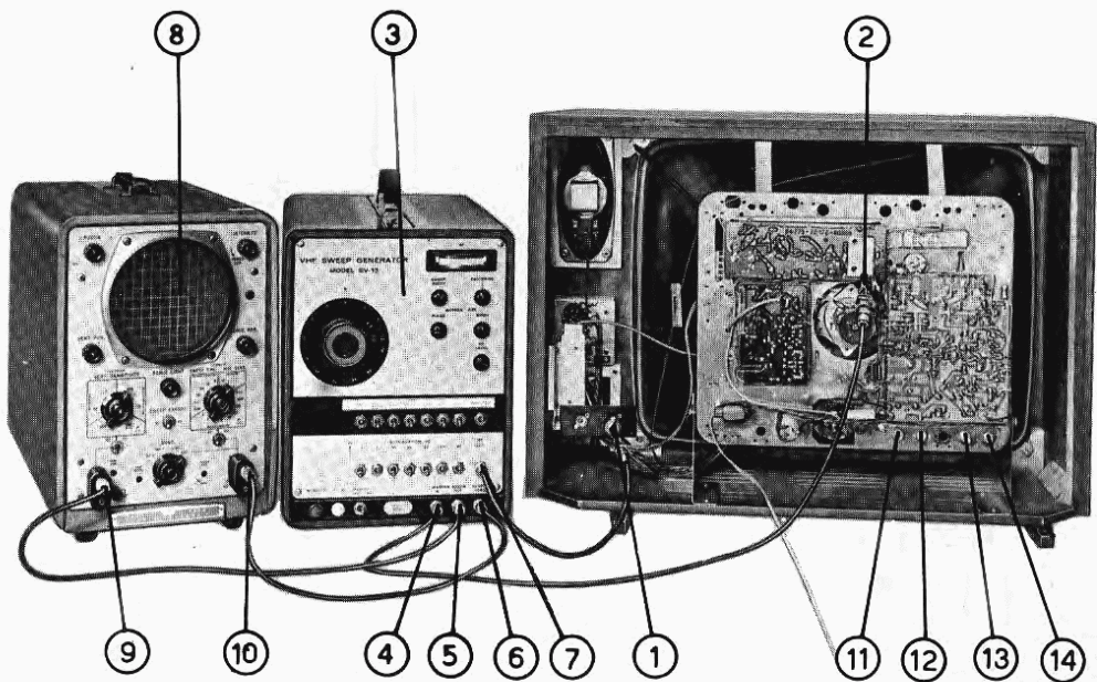
Fig. 5 - Disposizione degli strumenti per il controllo della copertura dei canali VHF.
