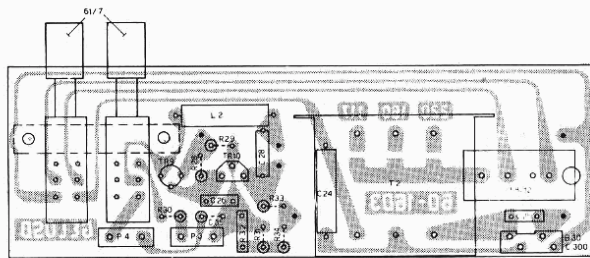
A sinistra: circuito stampato del sintonizzatore radio (G 6/81); sopra a destra: circuito amplificatore; sotto, circuito alimentatore e regolatore di velocità.
