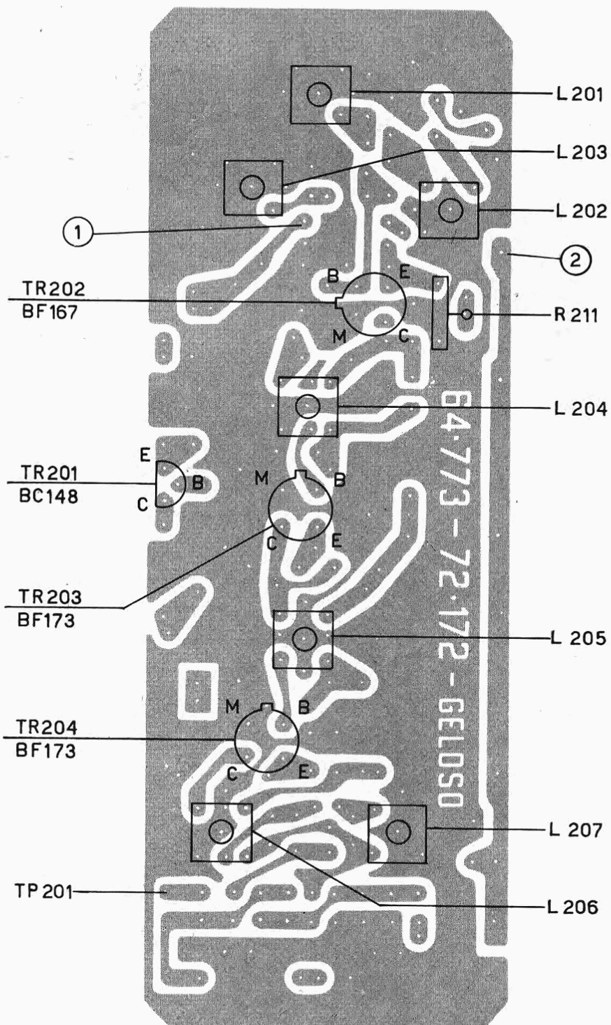
Fig. 2 - Piastra F.I. vista lato rame.
