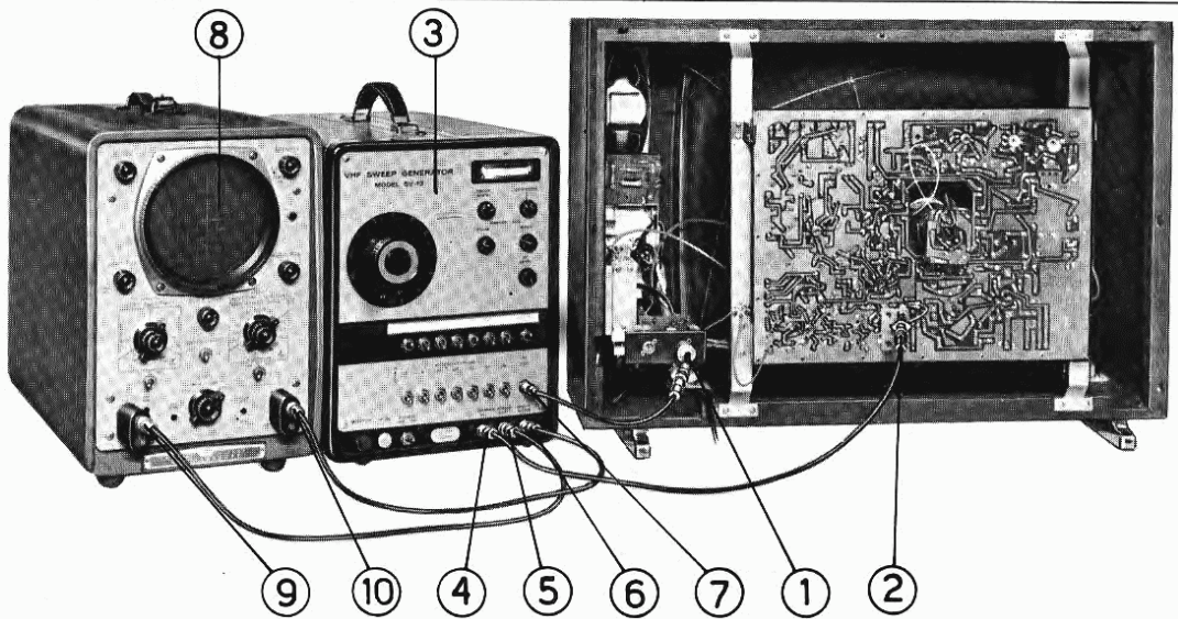
Fig. 12 - Disposizione degli strumenti per il controllo della copertura dei canali VHF con sintonizzatore a varicap.
