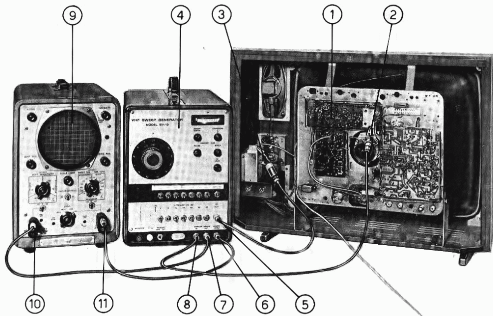
Fig. 1 - Disposizione degli strumenti per l'allineamento della sezione F.I.
