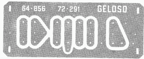
Piastrina gruppo A. F.
