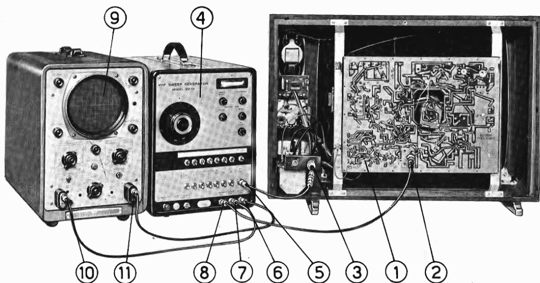
Fig. 8 - Disposizione degli strumenti per la messa in passo scala-frequenza
