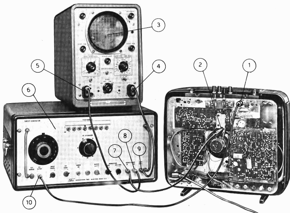
Fig. 6 - Disposizione degli strumenti per il controllo della copertura della banda UHF.
