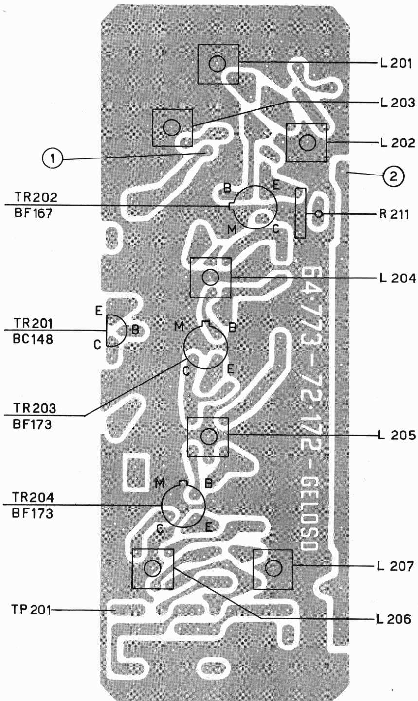
Fig. 2 - Piastra F.I. vista lato rame.
