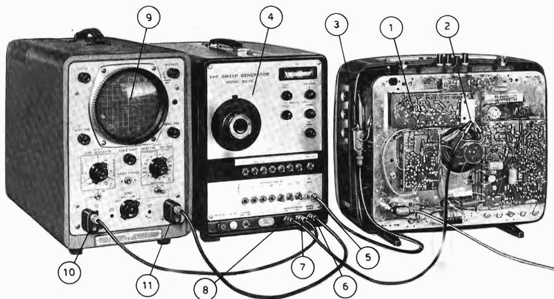
Fig. 1 - Disposizione degli strumenti per l'allineamento della sezione F.I.
