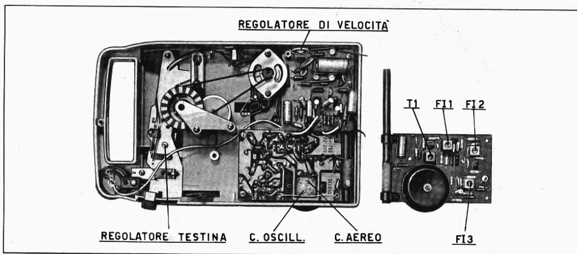
La figura mostra l'interno del lettore nastro G 19/123, e (a destra) il circuito radiorecettore dal lato componenti, coi riferimenti per la messa punto.
