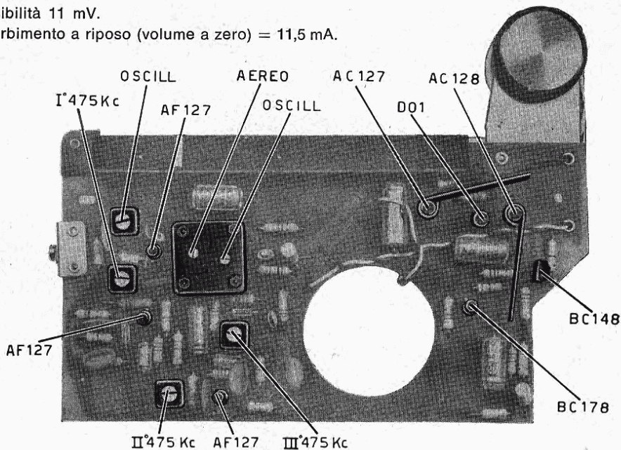
Circuito stampato del ricevitore G 16/250
