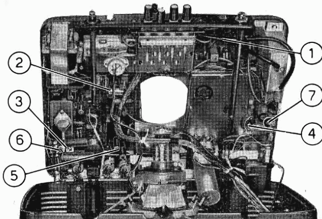
Fig. 8 - Vista superiore telaio
