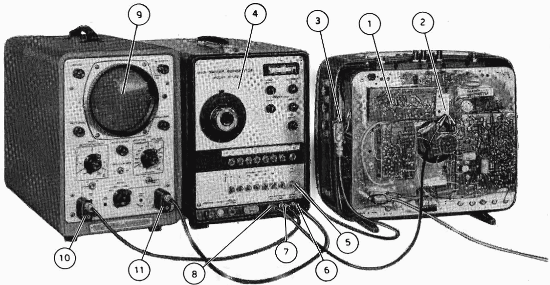
Fig. 1 - Disposizione degli strumenti per l'allineamento della sezione F.I.
