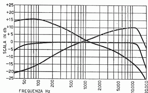
Curva di risposta dell'amplificatore G 1/190-TS Canale fono-radio.
