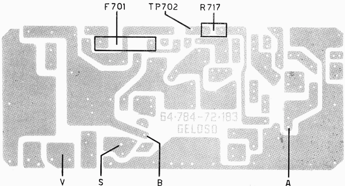
Fig. 4 - Piastra alimentazione vista lato rame.
