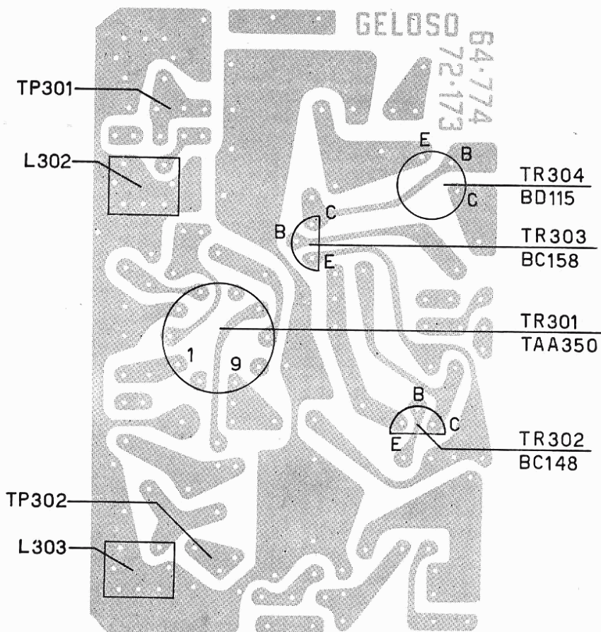
Fig. 9 - Piastra suono vista lato rame.
