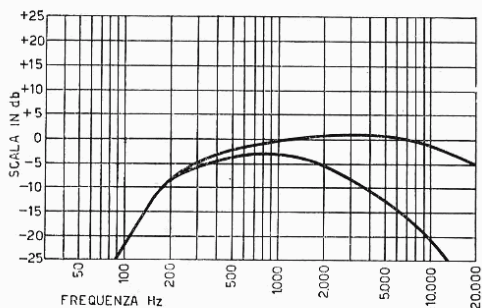
Curva di risposta (canali microfono) ed effetto della regolazione del controllo di tono.
