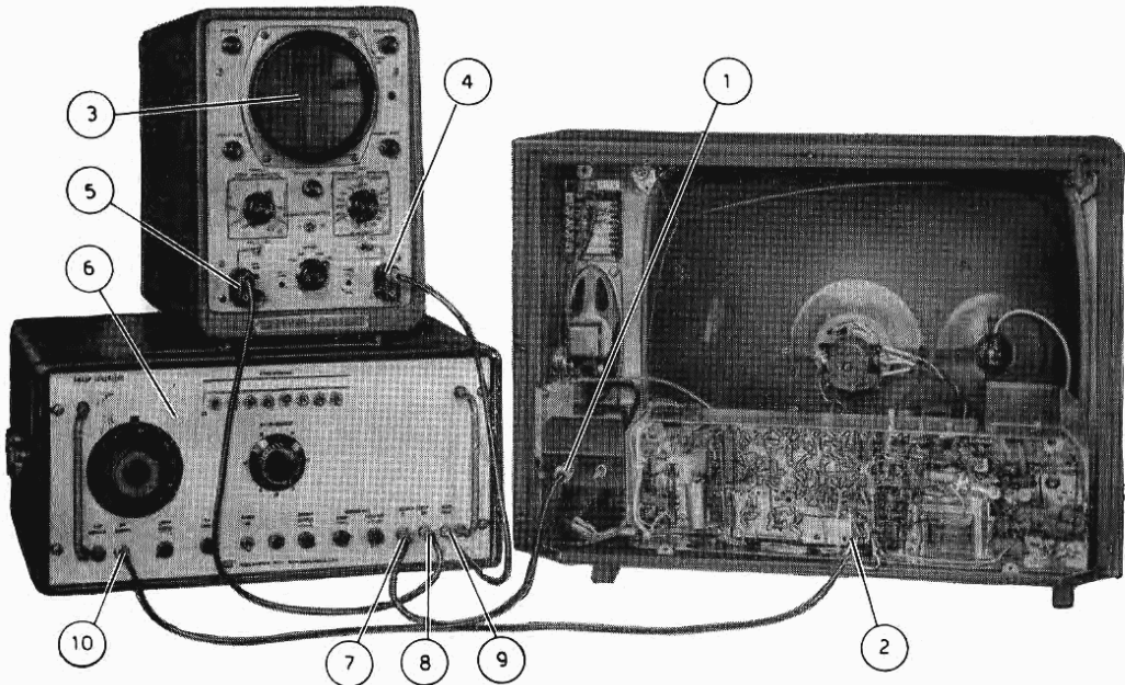
Fig. 7 - Disposizione degli strumenti per il controllo della copertura della banda UHF.
