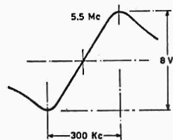
Fig. 8 - Fac-simile della curva di rivelazione del discriminatore a rapporto della sezione suono.
