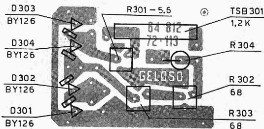
Circuito stampato alimentazione.
